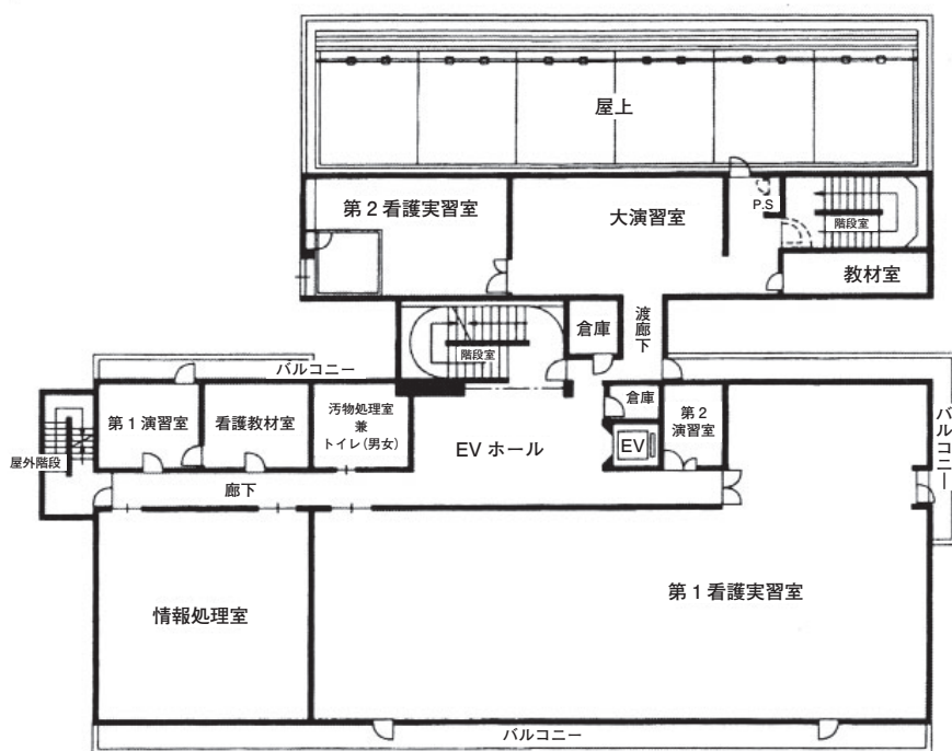
〈3 階平面図〉
