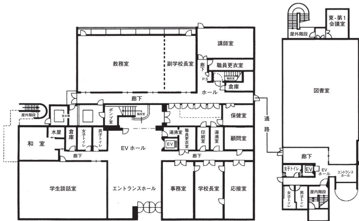
〈1 階平面図〉
