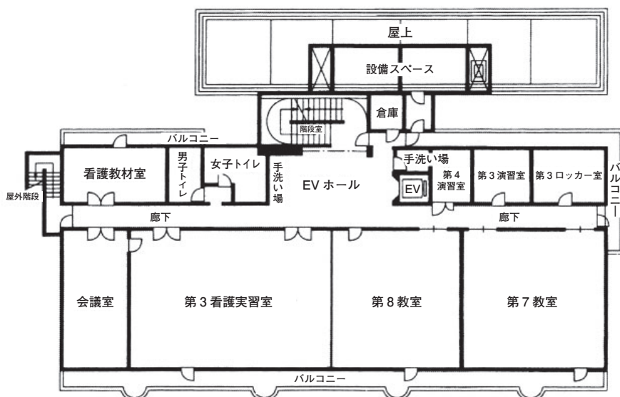
〈4 階平面図〉
